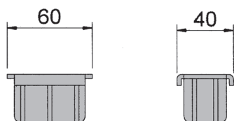
cod. 130004.00 tappo chiusura montante anteriore L=60 mm kg 0,015
