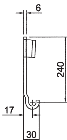
cod. 135013.20 * attacco standard cataforizzato kg 0,700
