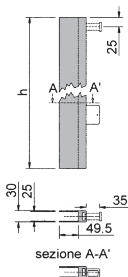
Laterale Side
