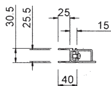
profilo X
