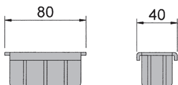
cod. 130003.00 tappo chiusura montante anteriore L=80 mm kg 0,025
