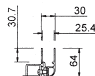
profilo Y
