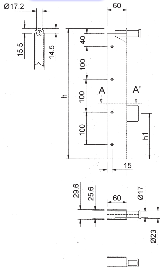
sezione A-A'
