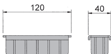
cod. 130005.00 tappo chiusura montan- te centrale posteriore kg 0,040
