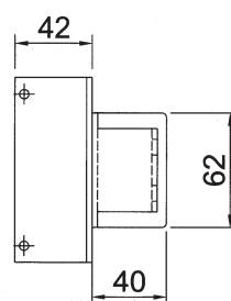
cod. 130007.01 taschetta con squadretta zincata a rivettare kg 0,300
