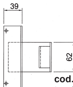
cod. 130006.00 taschetta a saldare kg 0,125 cod. 130006.01 taschette zincate kg 0,125
