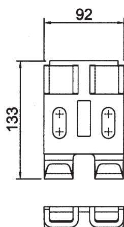
cod. 135013.20 * attacco standard cataforizzato kg 0,700
