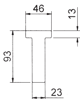
cod. 130073.00 attacco mobile per montante Italtop kg 0,190
